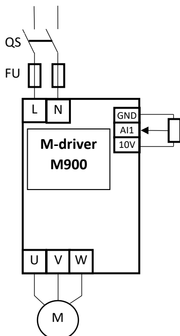
общий тип (M900-xxxG)
