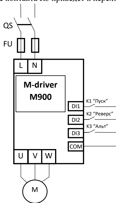
общий тип (M900-xxxG)
