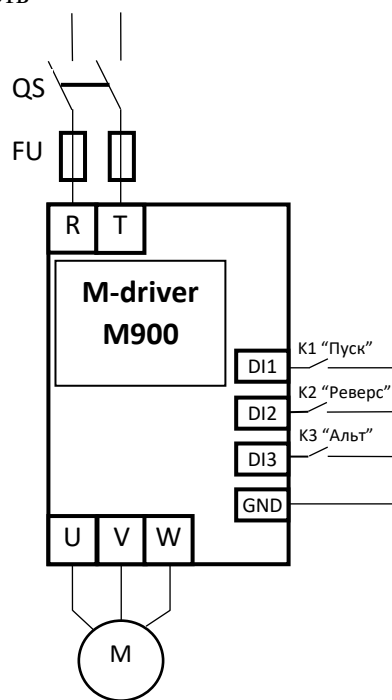
мини тип (M900-xxxM)
