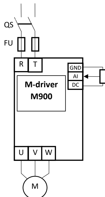
мини тип (M900-xxxM)
