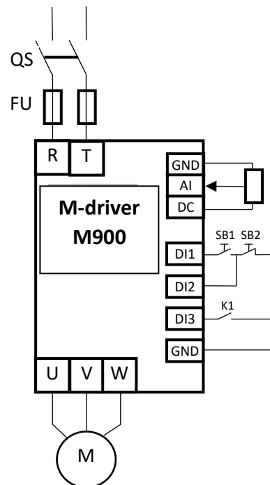
мини тип (M900-xxxM)
