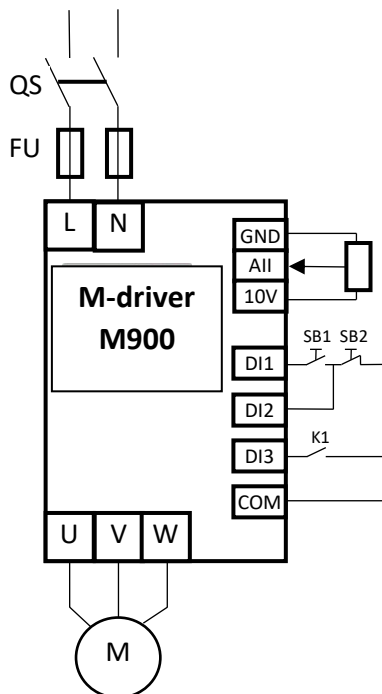
общий тип (M900-xxxG)
